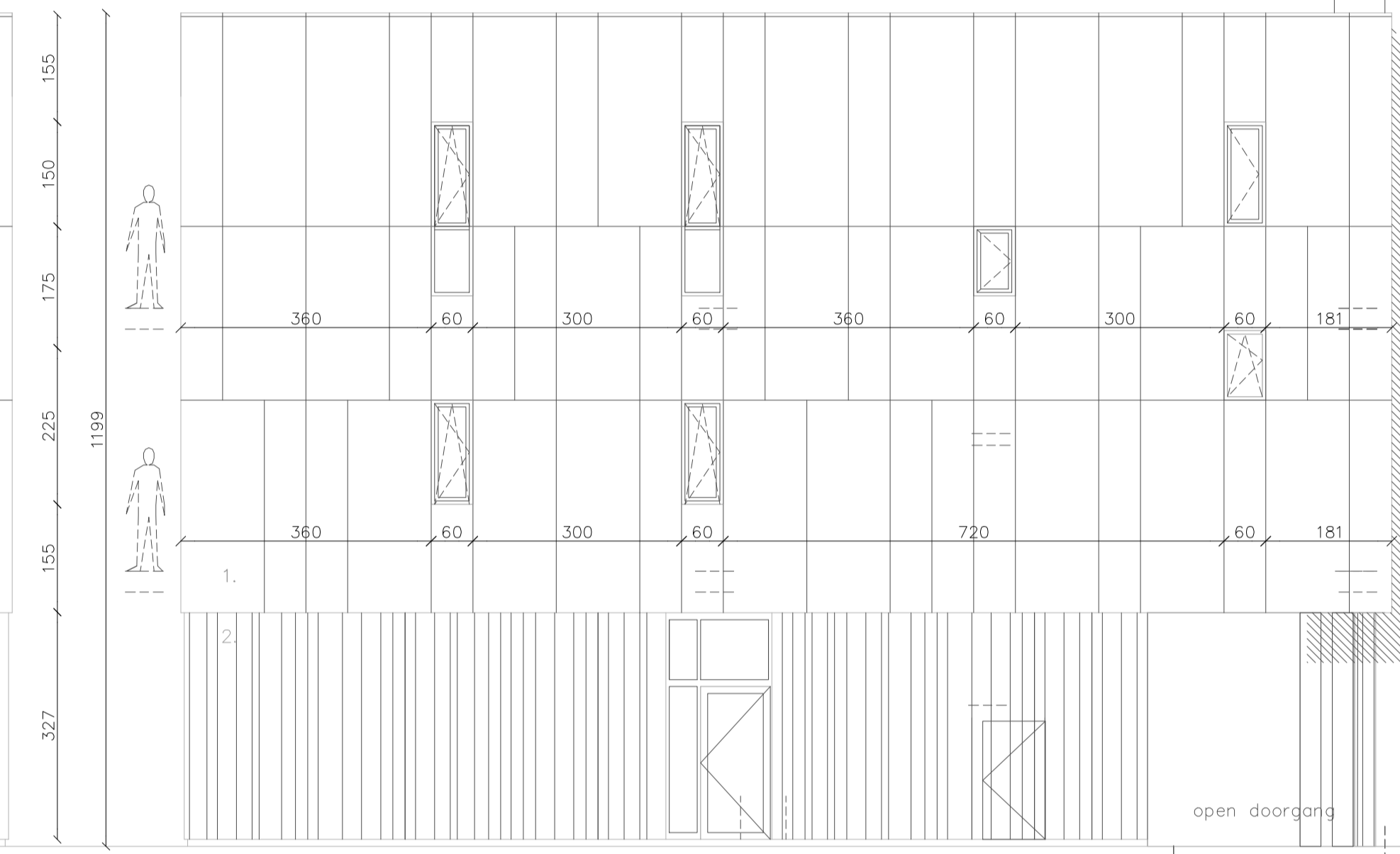
GEVEL NOORD
