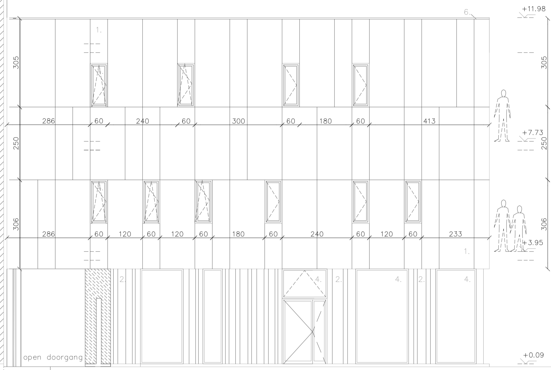
GEVEL ZUID
