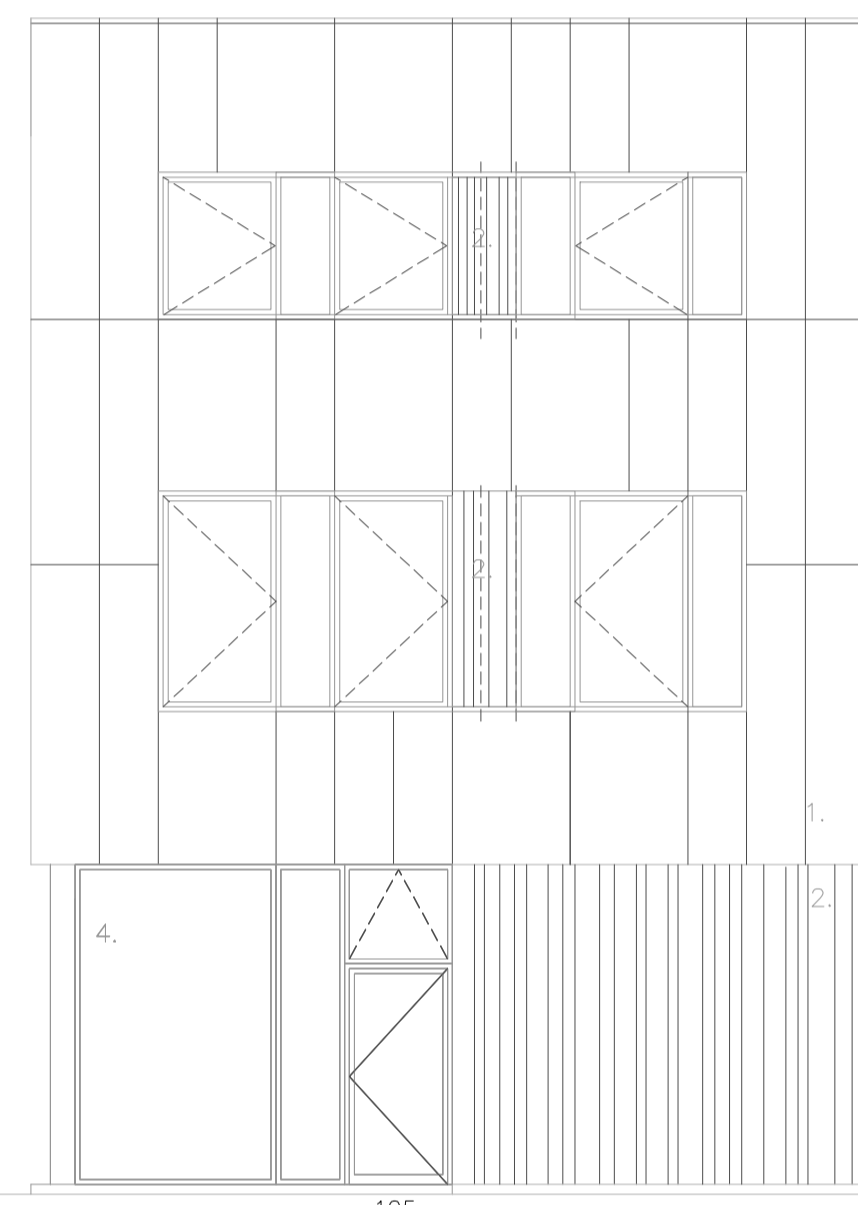
KOPGEVEL
